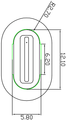
机板开孔尺寸
