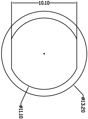
机板开孔尺寸
